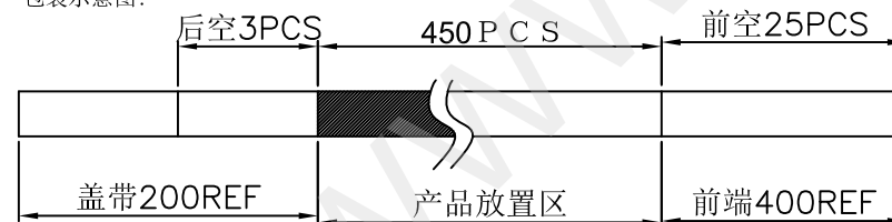
包装示意图:
