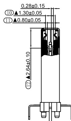
截面 A-A
